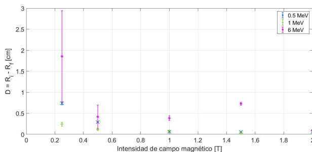
FIG. 4: Desplazamiento en la dirección radial de la trayectoria de electrones primarios, en función de la intensidad de campo magnético, para cada valor de energía cinética utilizada.
