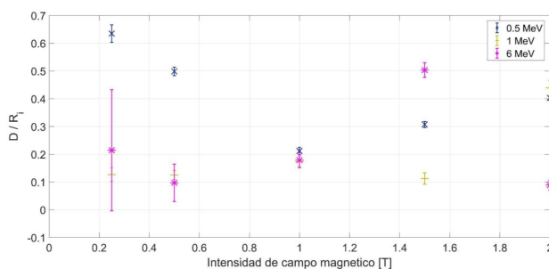
FIG. 5: Desplazamiento relativo al radio inicial de la trayectoria de electrones primarios, en función de la intensidad de campo magnético, para cada valor de energía cinética utilizada.
