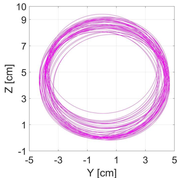
FIG. 2: Representación de la trayectoria del electrón, en presencia de campo magnético y con aire como medio dispersor. Caso de electrones de 6 MeV en campo de 0.5 T. Representación de la trayectoria del electrón, en presencia de campo magnético y con aire como medio dispersor. Caso de electrones de 6 MeV en campo de 0.5 T.
