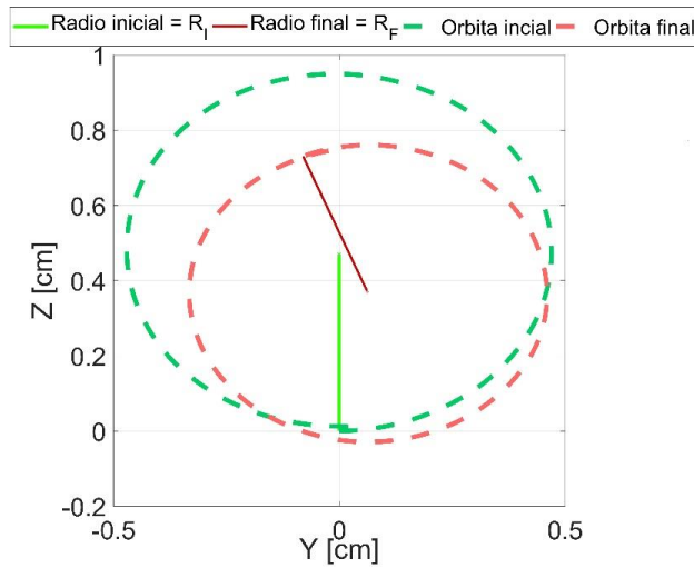
FIG. 3: Representación esquemática de las órbitas iniciales y finales de la trayectoria del electrón, en presencia de campo magnético y con aire como medio dispersor, con sus respectivos radios de curvatura.
