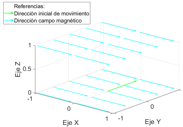
FIG. 1: Esquema simplificado de la configuración geométrica utilizada en las simulaciones Monte Carlo, para la caracterización de la trayectoria de electrones primarios en campo magnético externo uniforme.
