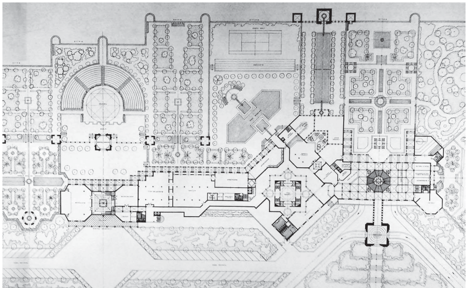
Figura 3: Proyecto Five Stars Hotel, Mosul, Iraq. Planta Baja. Repositorio: Fondo Chueca. Biblioteca de la E.T.S. de Arquitectura. Universidad Politécnica de Madrid (UPM).
