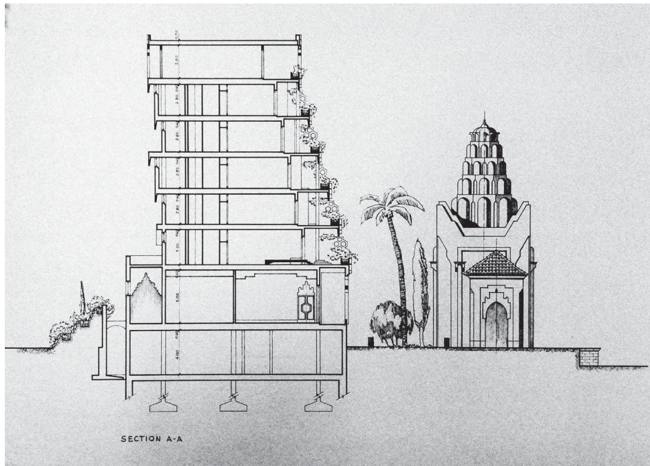
Figura 4: Proyecto Five Stars Hotel, Mosul, Iraq. Corte A-A. Repositorio: Fondo Chueca. Biblioteca de la E.T.S. de Arquitectura. Universidad Politécnica de Madrid (UPM).
