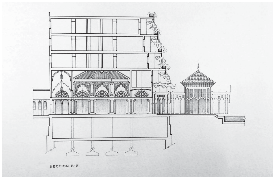
Figura 5: Proyecto Five Stars Hotel, Mosul, Iraq. Corte B-B. Repositorio: Fondo Chueca. Biblioteca de la E.T.S. de Arquitectura. Universidad Politécnica de Madrid (UPM).
