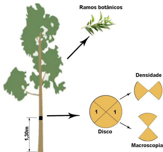
Fig. 1. Esquema de amostragem e localização das amostras para identificação botânica, massa específica e caracterização macroscópica.
