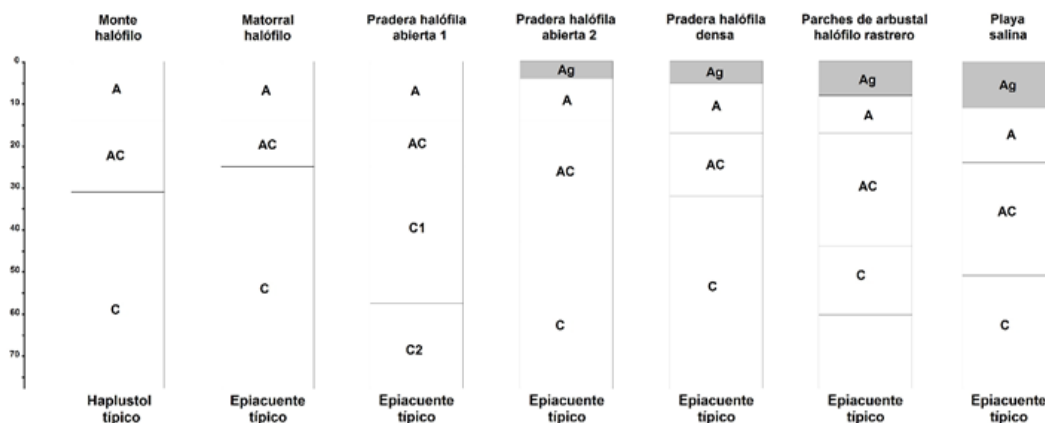
Figura 7. Morfología de los perfiles de la segunda zona de muestreo (profundidad en cm).
