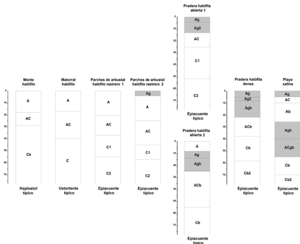
Figura 6. Morfología de los perfiles de la primera zona de muestreo (profundidad en cm).
