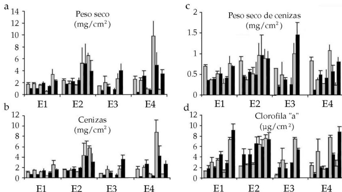
Figura 5. Variables del perifiton registradas desde enero a octubre de 1999 en cada estación de muestreo. a: peso seco; b: cenizas; c: peso seco libre de cenizas; d: clorofila 'a'. (barra = DS = \pm 1 ). Para cada estación de muestreo las barras de izquierda a derecha se corresponden con los meses de enero a octubre respectivamente.
