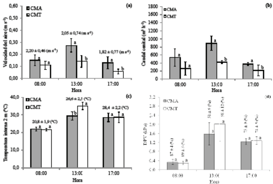
Figura 3. Efecto de los invernaderos ‘Capilla Modificado Alternativo’ (CMA) y ‘Capilla Modificado Tradicional’ (CMT) sin cultivo sobre la velocidad del aire ( m s^{-1} ), caudal en las ventanas cenitales ( m^3 h^{-1} ), temperatura interna ( ^{\circ}C ) y déficit de presión de vapor, DPV (kPa) en la fase experimental 1. Las líneas en cada barra representan el desvío estándar. Los valores sobre cada barra en las figuras (a) y (c), representan la media y el desvío estándar de cada factor en el ambiente externo a los invernaderos, y en la figura (d) la humedad relativa externa. Letras diferentes en cada hora representan diferencias estadísticas según el test de Tukey ( P \leq 0,05 ).
