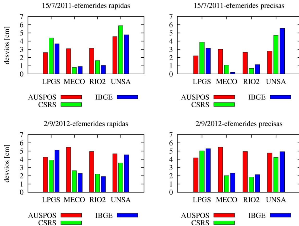
Figura 6: MDES obtenido para los tres servicios, según el tipo de efemerides. Se consideraron archivos de 12 hs de observación correspondientes a los días 15/7/2012 (superior) y 2/9/2012 (inferior).
