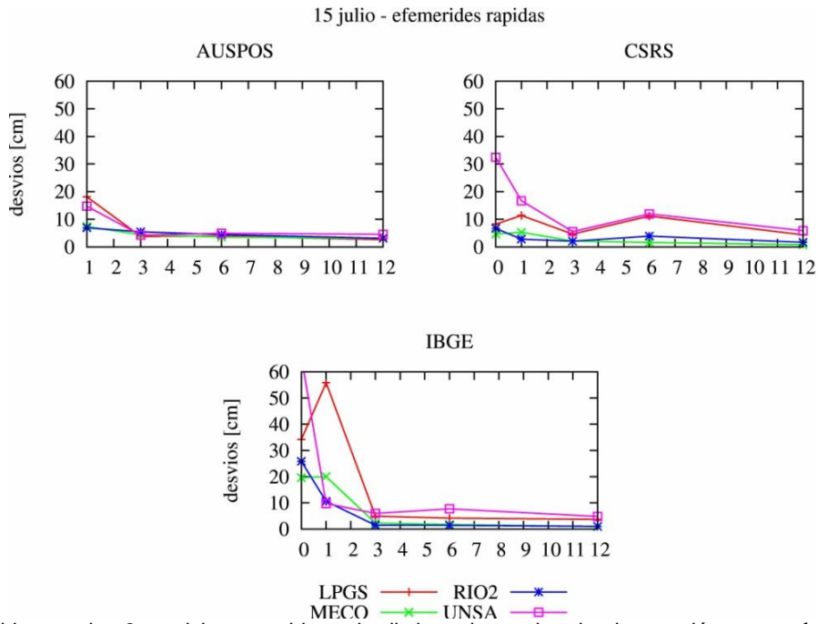
Figura 5: MDES obtenido para los 3 servicios, considerando distintos intervalos de observación y con efemérides rápidas. Luego de las 6 horas de medición, no se evidencian diferencias apreciables con los obtenidos utilizando efemérides precisas.
