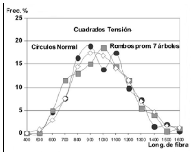
Figura N° 4 (Árbol 2) Distribución de frecuencias de longitudes de fibra
