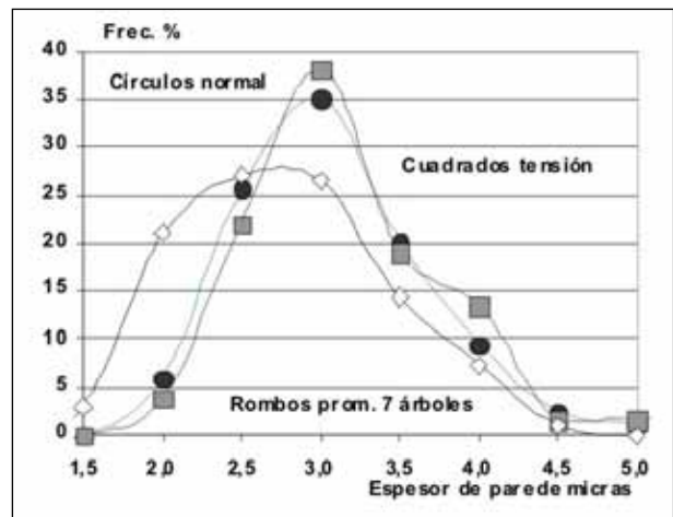
Figura N° 8 (Árbol 2) Distribución de frecuencias de espesores de pared de fibra
