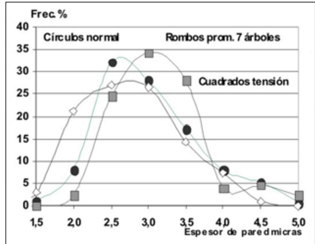
Figura N° 7 (Árbol 1) Distribución de frecuencias de espesores de pared de fibra
