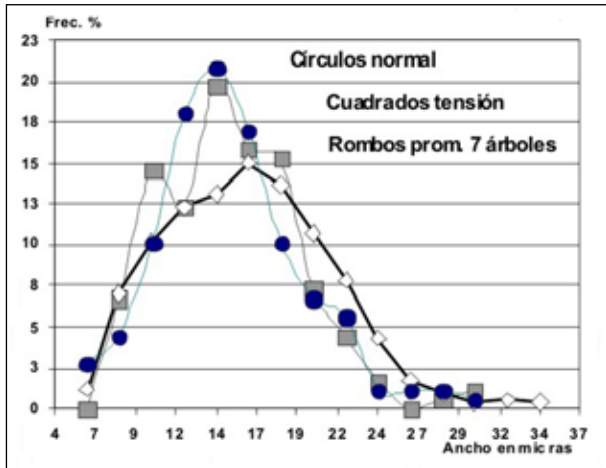
Figura N° 5 (Árbol 1) Distribución de frecuencias de anchos de fibra
