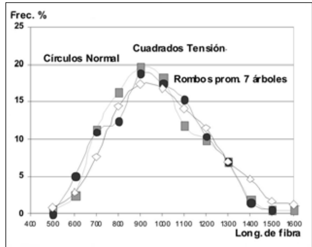
Figura N° 3 (Árbol 1) Distribución de frecuencias de longitudes de fibra
